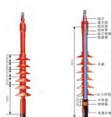
35kV单芯户外终端安装图
