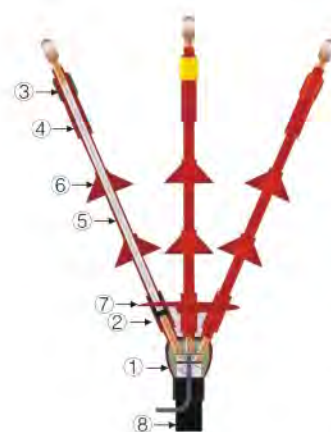
10kV三芯热缩终端剖面图
